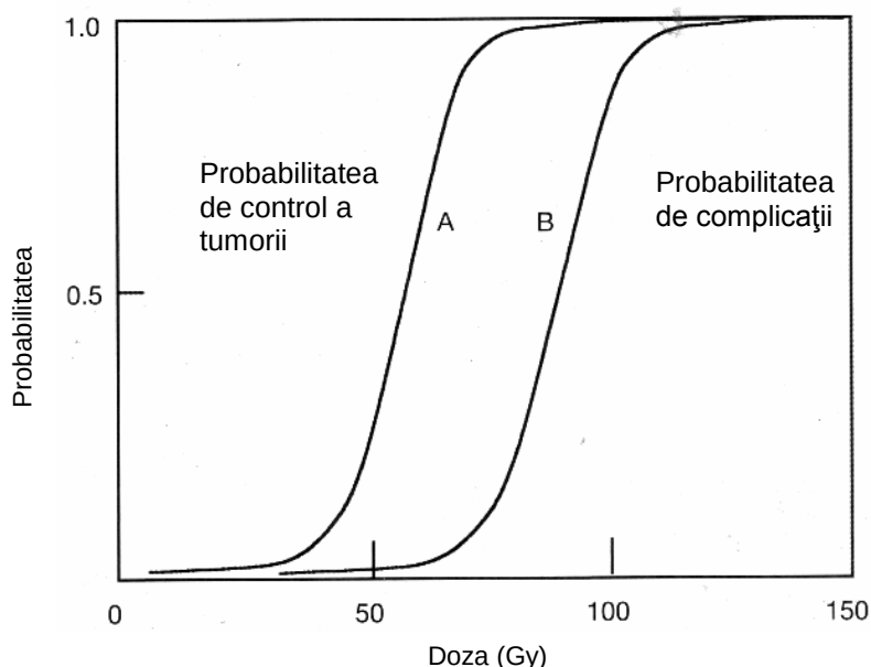
Principiul randomamentului terapeutic. Curba A reprezintă TCP, iar curba B reprezintă NTCP
